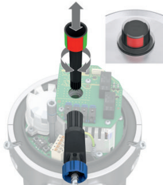
Bild 20: Stellungsanzeige über Anzeigewelle voreinstellen
