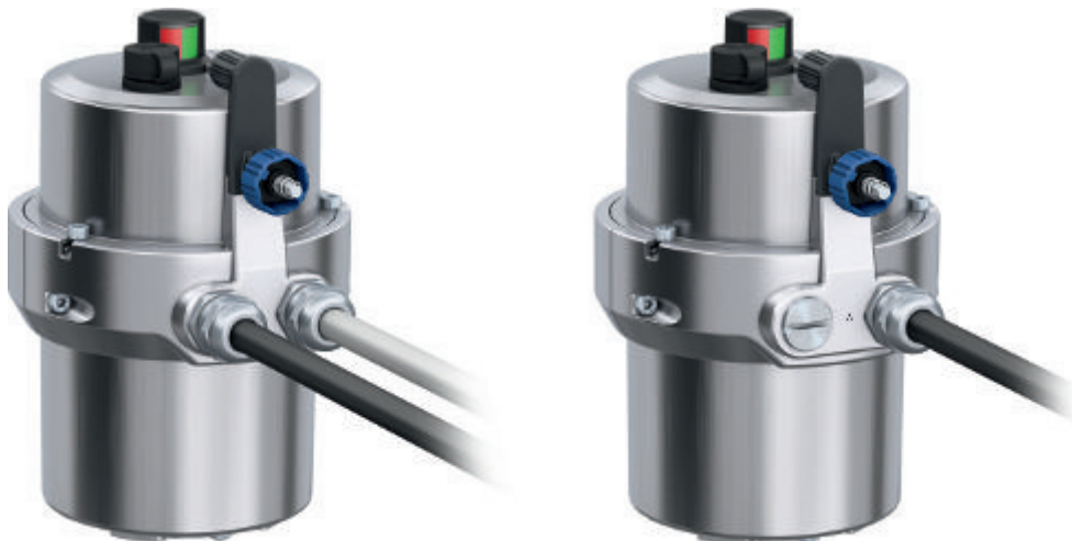
Bild 4: Kabeleinführung bei zwei Leitungen und bei einer Leitung
