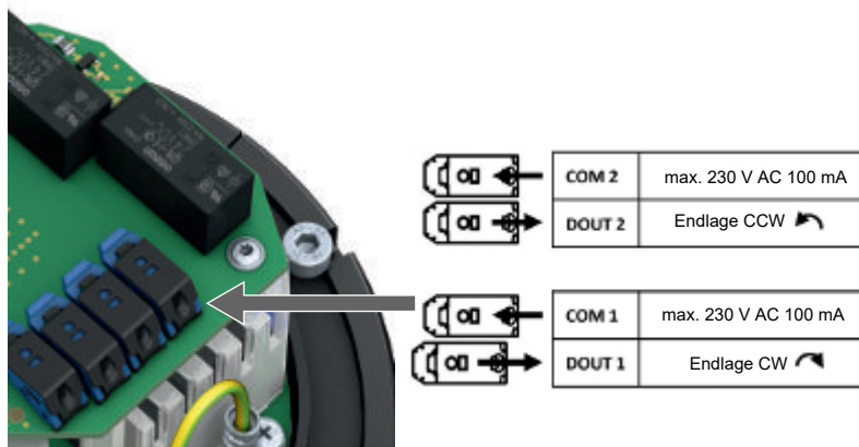
Bild 9: Steckklemmen Option 2, Multi I/O Modul
