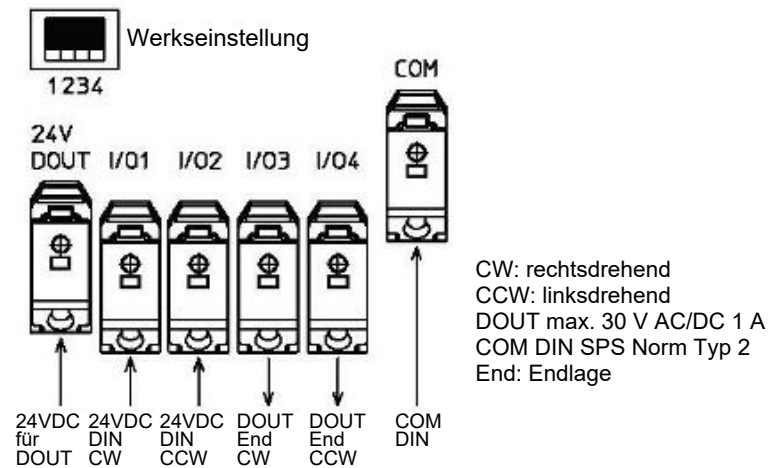
Bild 16: Ein- Ausgangsbelegung bei Werkseinstellung
