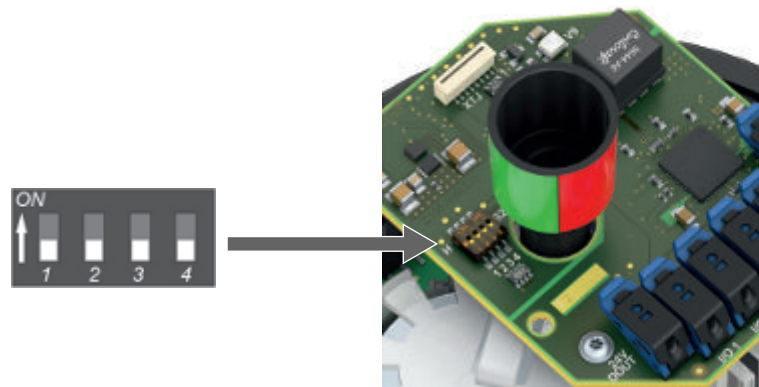
Bild 15: DIP-Schalter S2 für Multi I/O Modul
