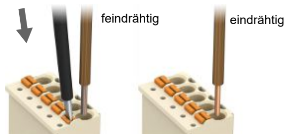
Bild 6: Leitungen an Steckklemmen anschließen
