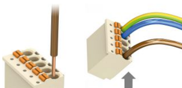
Bild 7: Federleiste abziehen
