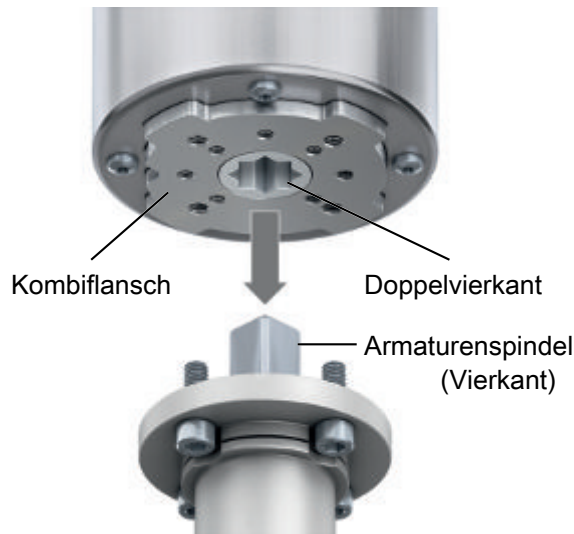
Bild 2: Stellantrieb aufsetzen
