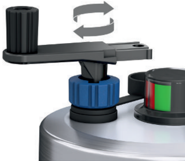
Bild 18: Stellantrieb/Armatur im Handbetrieb betätigen
