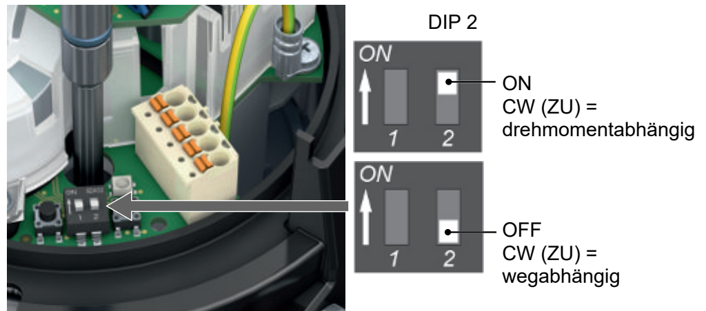
Bild 12: Abschaltart über DIP-Schalter 2 einstellen
