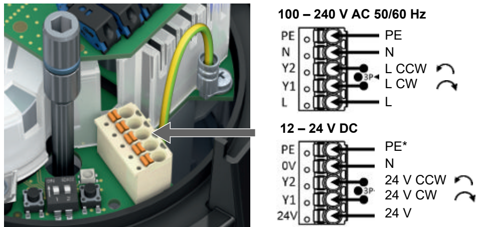
Bild 5: Federleiste mit Steckklemmen (Bild zeigt Grundauführung, Leistungsklemmen)
